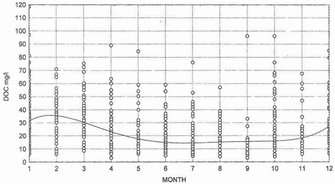
Figure 1e. High Range DOC Subarea Monthly DOC
