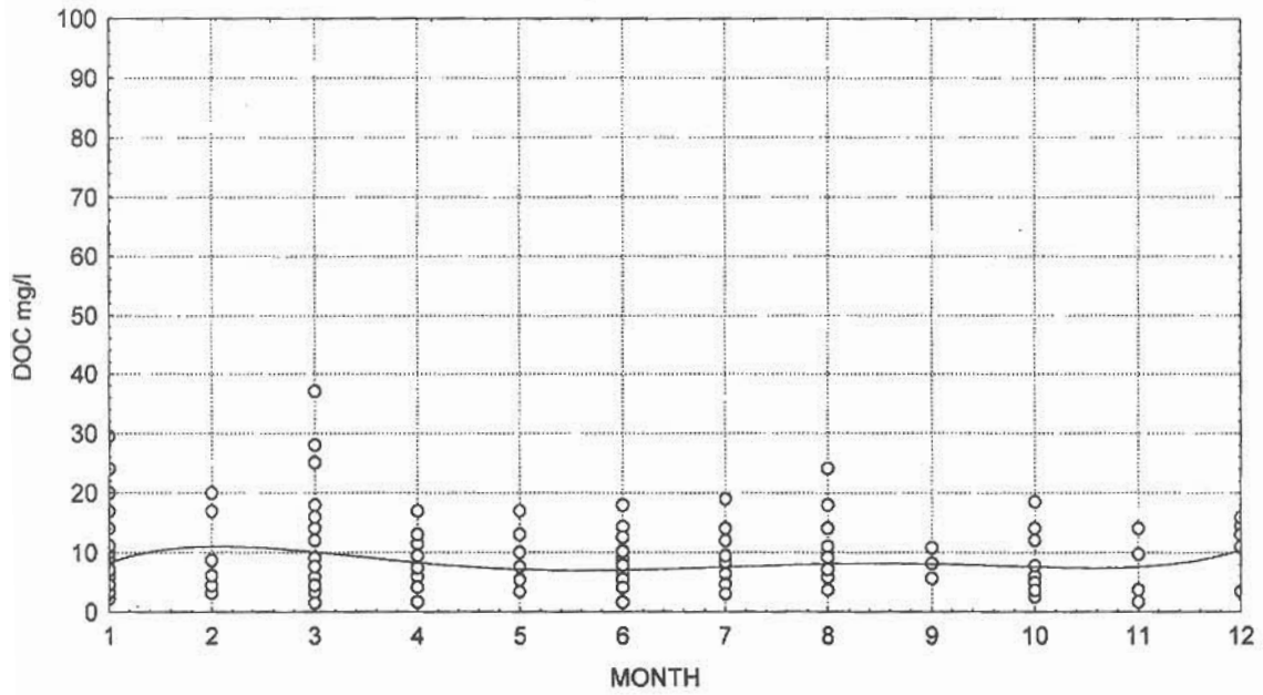
Figure 1c. Midrange DOC Subarea Monthly DOC
