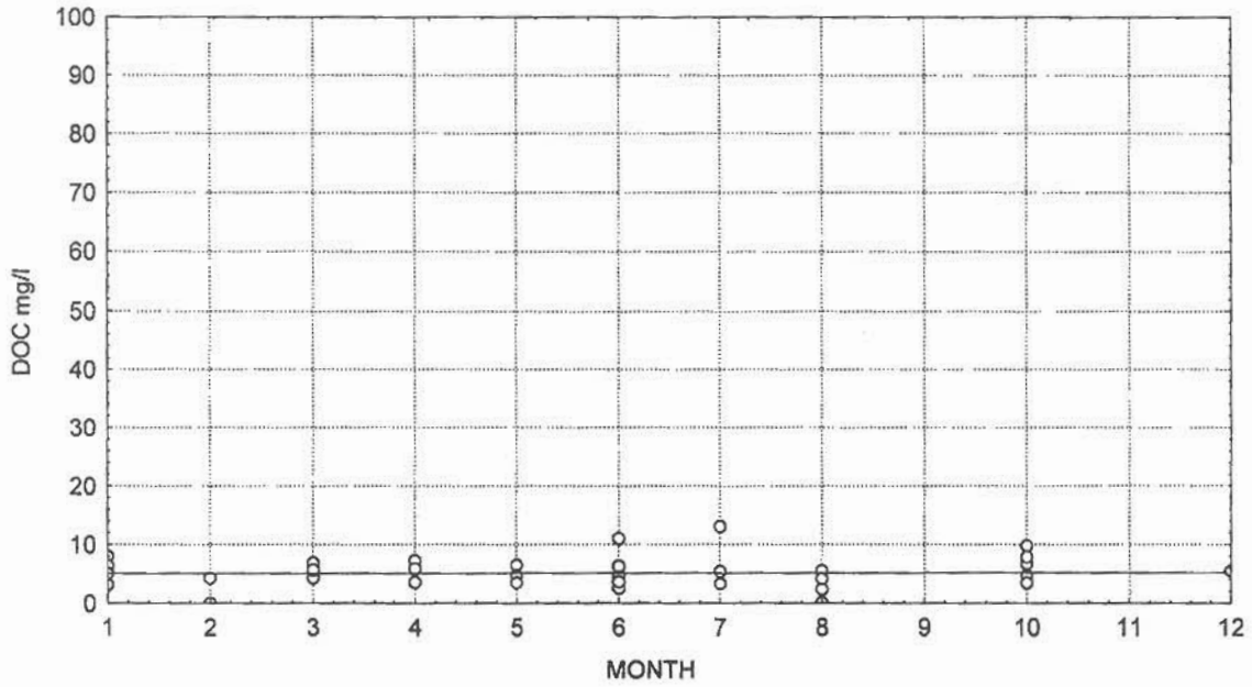
Figure 1a. Low Range DOC Subarea Monthly DOC
